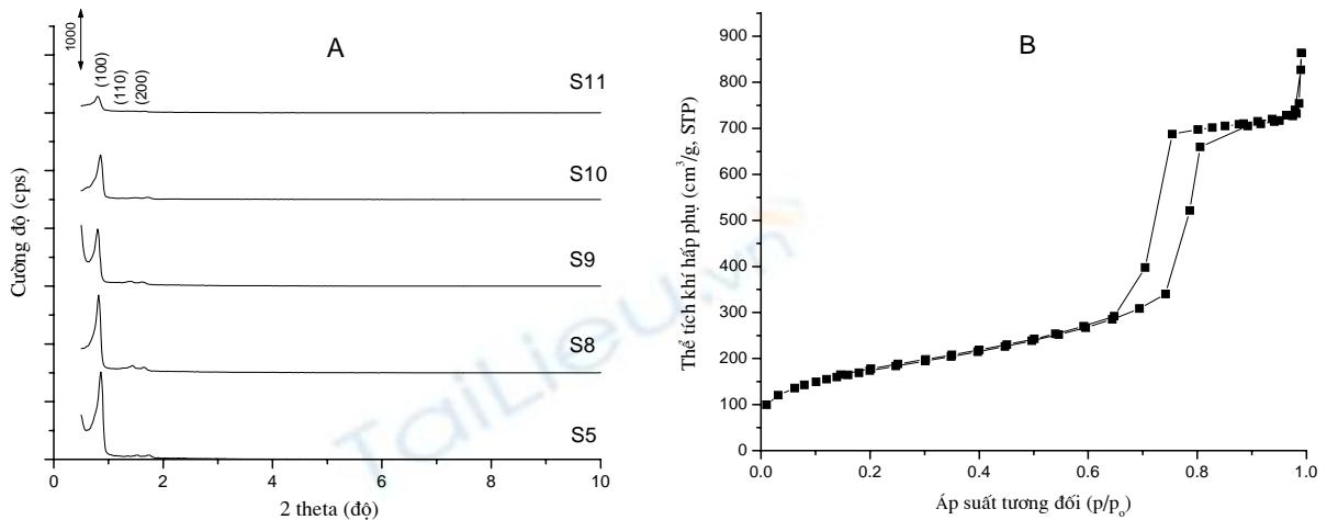
Hình 3: (A) Ảnh hưởng của tỉ lệ \text{H}_2\text{O}/\text{TEOS} đến sự tạo thành pha mao quản trung bình lục lăng; (B). Đường đẳng nhiệt hấp phụ-giải hấp phụ đẳng nhiệt nitơ của mẫu S5
