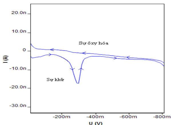
Hình 1. Đường cong dòng thế tuần hoàn (CV) của 0,05 mg/l \text{DMDSe} trong nền \text{CH}_2\text{Cl}_2/\text{C}_2\text{H}_5\text{OH} (1/1) + HCl 0,06 M + \text{LiClO}_4 0,2 M Tốc độ quét thế 50 mV/s.
