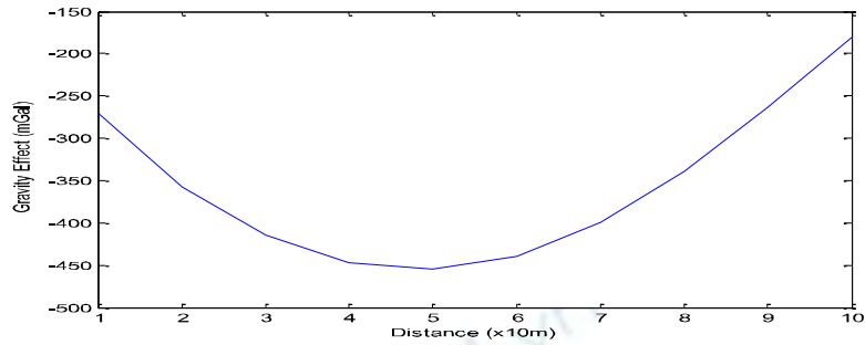
Hình 10. Đồ thị độ thường trọng lực do mặt móng kết tinh gây ra trên mặt đất
