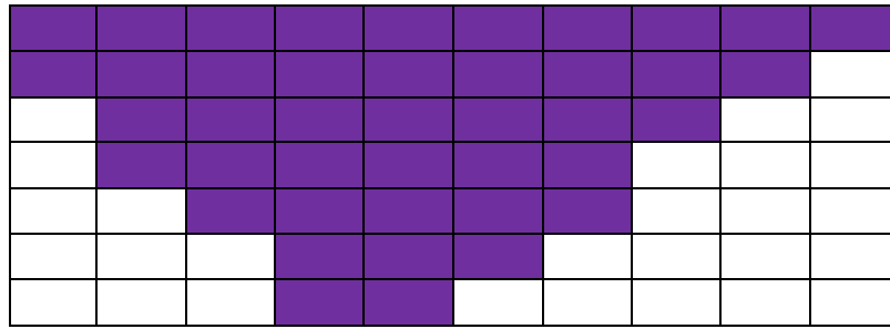
Hình 9. Mô hình mặt móng bồn trầm tích thứ ba.
