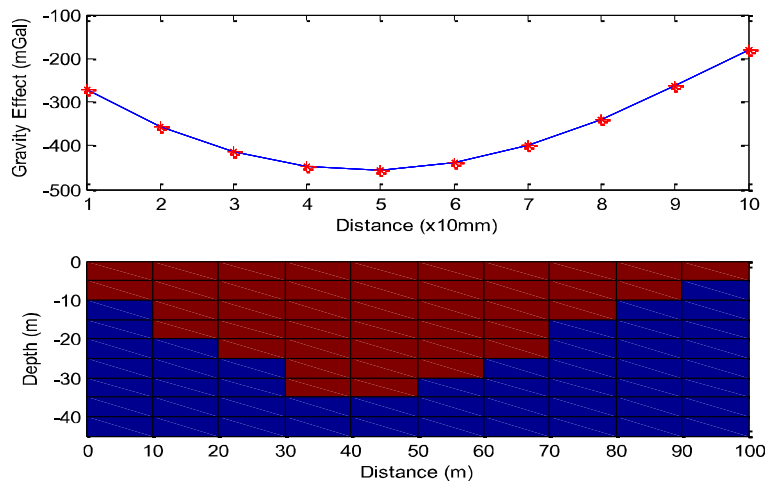
Hình 12. Đồ thị độ thường trọng lực được tính toán lại và địa vật được tìm thấy sau lần lặp thứ 800 của phương pháp compact
