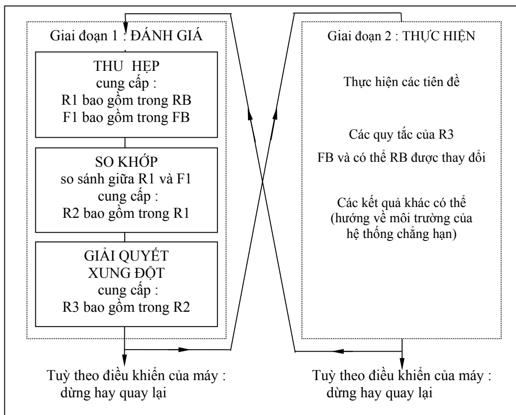
Hình 3.1 Chu kỳ cơ bản của một máy suy diễn
