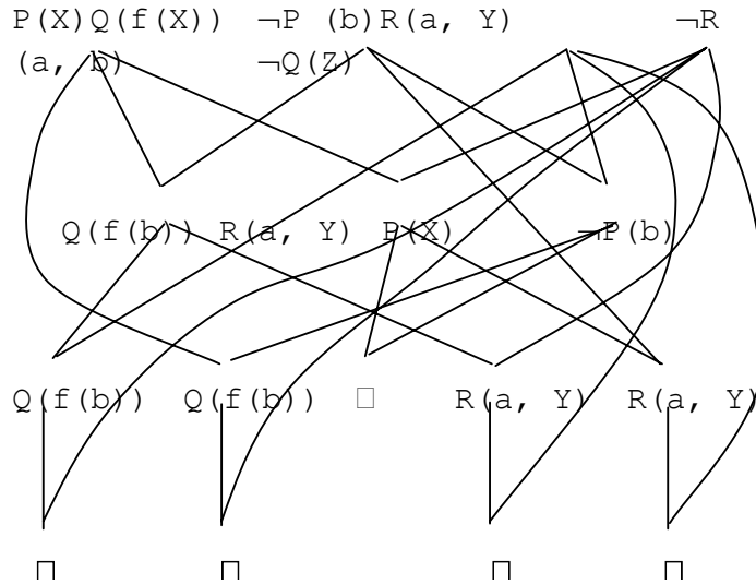
Hình 2.4. Đồ thị định hướng
