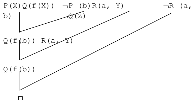
Hình 2.5. Đồ thị bác bỏ
