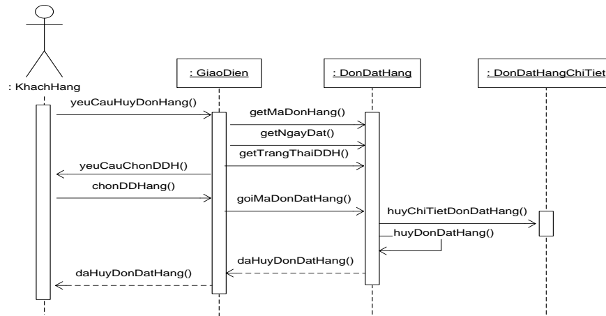
Biểu đồ tuần tự của user – case đặt hàng
