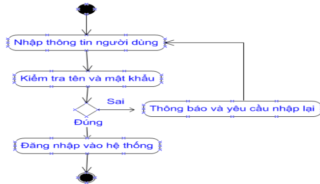
Biểu đồ hoạt động của user – case đăng nhập
