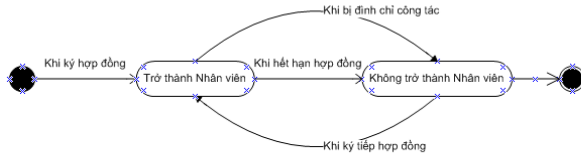
Biểu đồ trạng thái lớp: NHÂN VIÊN
