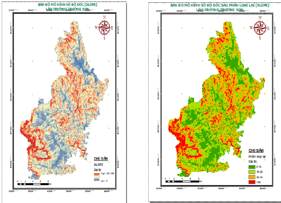
Hình 4. Kết quả xây dựng mô hình số độ dốc trước và sau phân loại lại.
